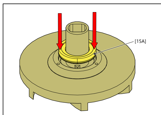
Fig. 3.4.9 Drücken Sie gleichzeitig mit beiden Händen den statischen Teil [15A] der Gleitringdichtung bis zum Ende.
