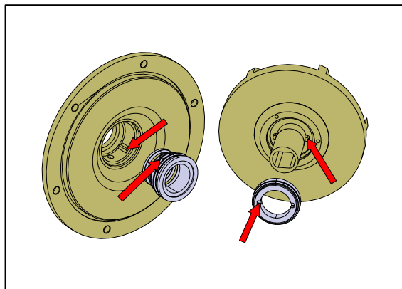
Fig. 3.4.5 Beim Einsetzen der Gleitringdichtung sind Verzahnungen im hinteren Gehäuse [12] und Laufrad [90] sowie Einschnitte in der Gleitringdichtung vorhanden. Richten Sie sie aus, um eine ordnungsgemäße Montage zu gewährleisten.
