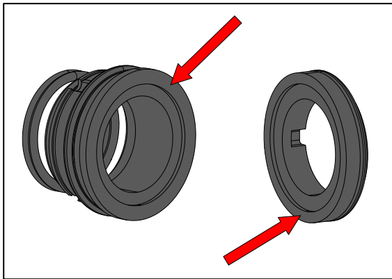
Fig. 3.4.4 Dichtflächen sorgfältig reinigen und entfetten.
