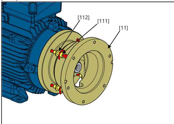
Fig 3.3.11 Entfernen Sie die Schrauben [111] und Unterlegscheiben [112], mit denen die hintere Abdeckung [11] am Motor befestigt ist.
