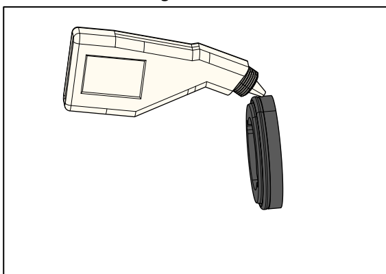
Fig. 3.4.8 Schmieren Sie den rotierenden Teil [15A] der Gleitringdichtung, um eine genauere Montage zu gewährleisten. Verwenden Sie eine schnell
