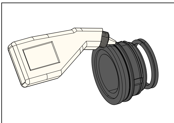
Fig. 3.4.6 Schmieren Sie den statischen Teil [15B] der Gleitringdichtung. Verwenden Sie eine schnell verdunstende Flüssigkeit wie Alkohol.
