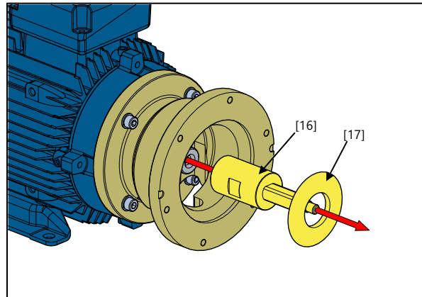
Fig 3.3.10 Entfernen Sie die Welle [16] mit dem Abweiser [17].
