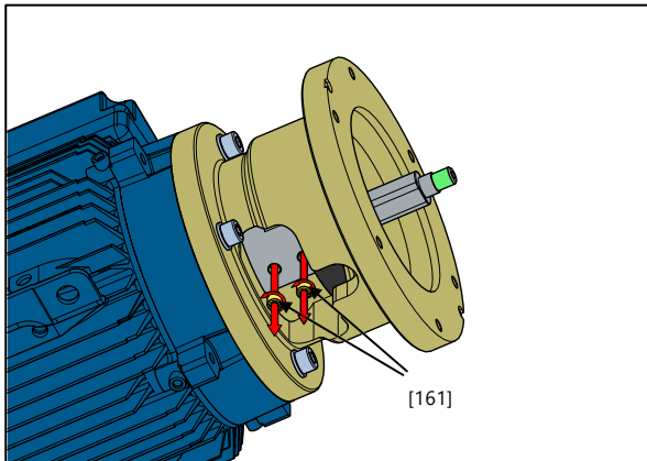
Fig 3.3.9 Lösen und entfernen Sie die Sicherungsschrauben [161].
