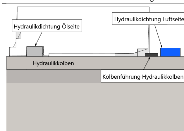
Fig 3.9.1 FP/FH 25 Dichtungsanordnung.
