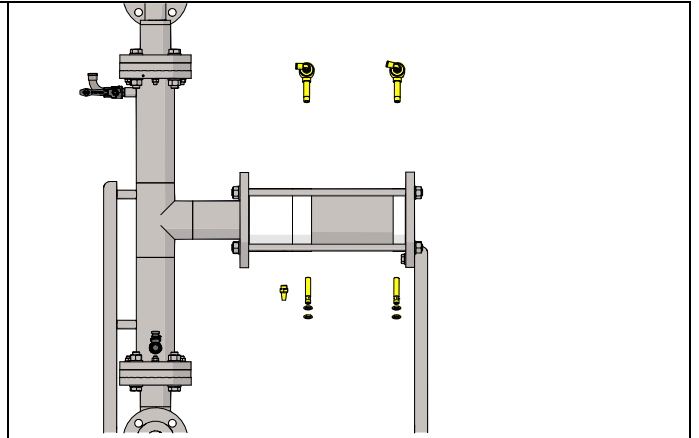
Fig. 3.6.3d Entfernen Sie die Schnellauslassventile [32], Sensoren [30] und Bronzeschalldämpfer [63]. Entfernen Sie den Sensor jedoch nur, wenn nötig
