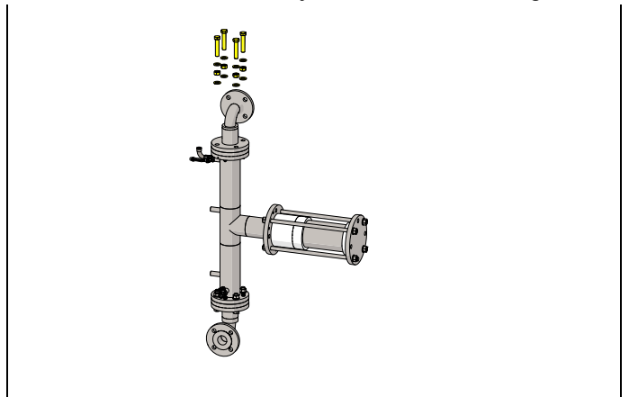
Fig. 3.6.5a Lösen und entfernen Sie acht Sechskantschrauben [38], die den Druckstutzen [3] mit den Gehäusen [1] verbinden.
