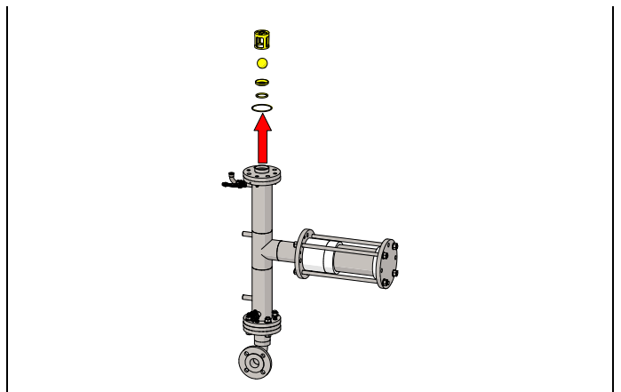
Fig. 3.6.5c Entfernen Sie die Kugelfänge [11], die Ventilkugeln [20], die Ventilsitze [19], die O-Ringe, den Ventilsitz [16] und den O-Ring Flansch [24] von den Gehäusen [1].
