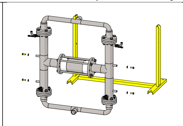
Fig. 3.7.5a Lösen und entfernen Sie acht Sechskantschrauben [38], die den Druckstutzen [3] mit den Gehäusen [1] verbinden.
