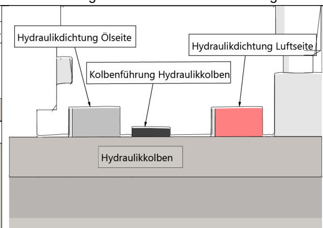
Fig 3.9.2 FP/FH 40-80 Dichtungsanordnung.
