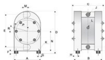
Standardpumpe PE
