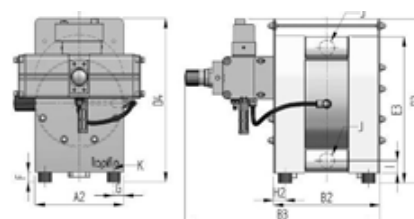
Filterpresspumpen TF
