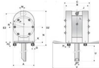
Fasspumpen TD
